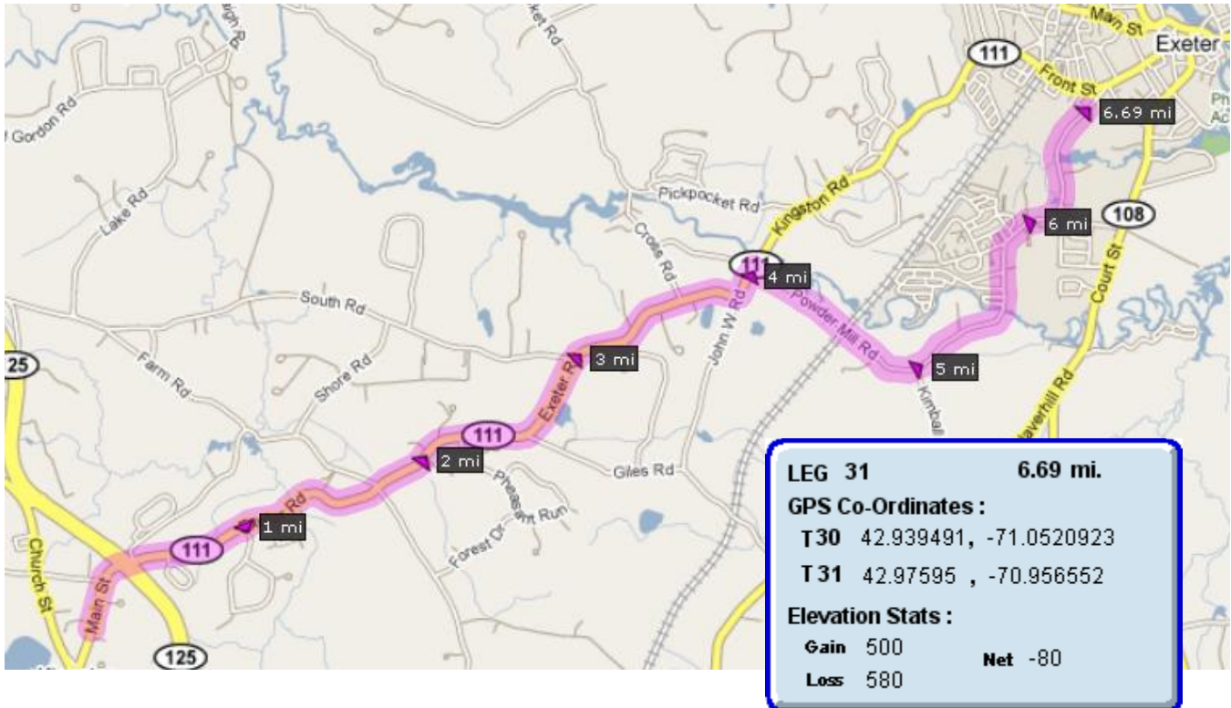
RTB2009: Leg 31
