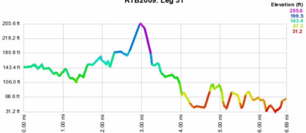
RTB2009: Leg 31
