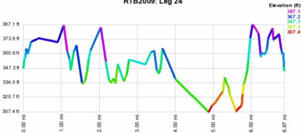
RTB2009: Leg 24
